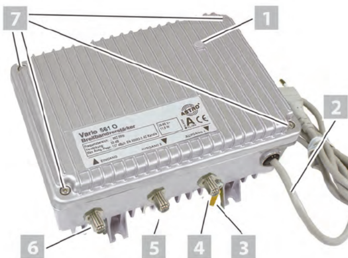
Bild 1: Verstärker VARIO 561 O (VARIO 662, VARIO 683 O u. VARIO 684 O ähnlich) VARIO 561 PG11 O ist mit PG11 Gewindeanschlüssen ausgestattet
