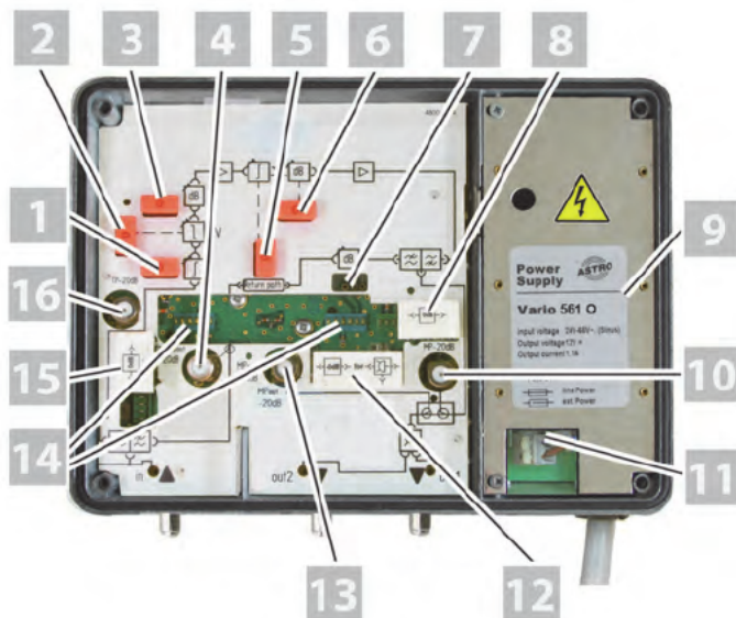
Bild 2: Verstärker VARIO 561 O, innen (VARIO 662 O, VARIO 683 O u. VARIO 684 O ähnlich) VARIO 561 PG11 O ist mit PG11 Gewindeanschlüssen ausgestattet
